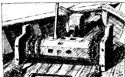
8. Bråspel, "spakspel", på jakten "Njord" från Korpo. Spelet nybyggt år 1933 -. Det tidigare spelet, byggt samtidigt som jakten omkr. år 1900, hade spelnockar utanför betingarna och i dessa hål för spakarna. (Pall av järn).
