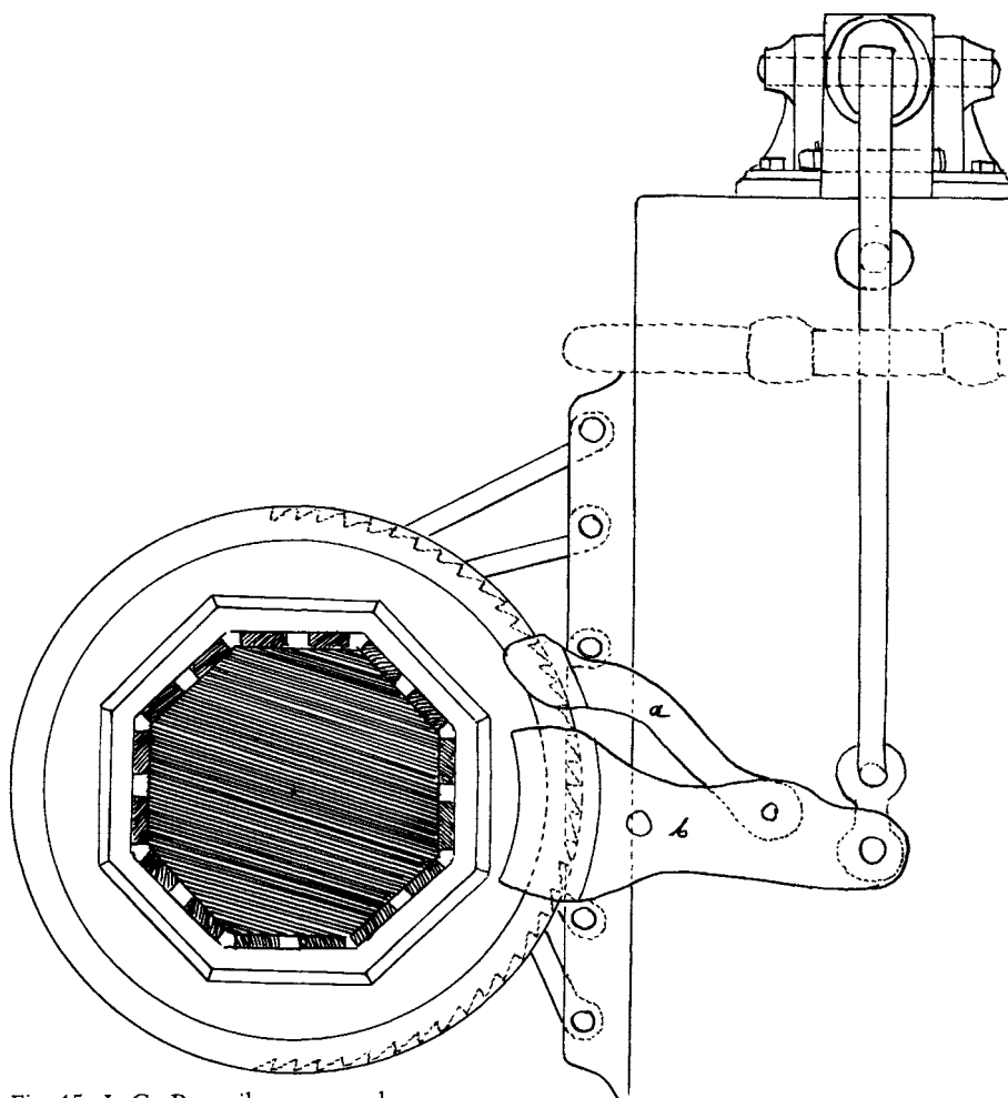
Fig. 15. J. G. Bergviks pumpspjel.
