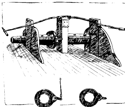
11. Pow & Fawcus' pumpspel sett förifrån.
