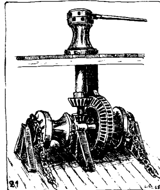
21. Emerson & Walkers ankarspel
