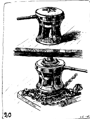
20. Gångspel från seglande örlogsfartyg, "barbotinspel". 1800-talet.
