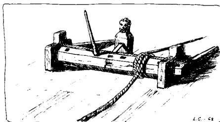
5. Vindspel - bråspel - på engelsk pink från slutet av 1600-talet. (efter Rålamb.)
