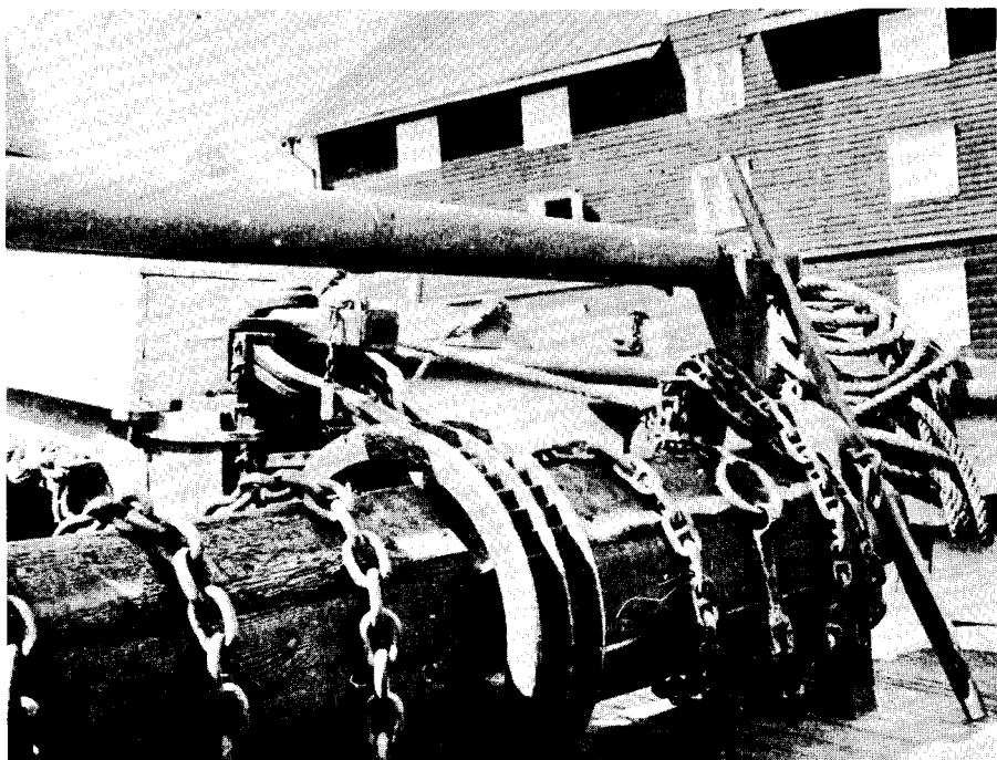
Bild 13. Spelet på galeasen NORDEN av Källvik. Tillhörde först en gammal öregrundsskuta HELMI, som ägdes av NORDENS redare Pettersson. HELMI högs upp 1906 och Pettersson skiftade då spelet över till NORDEN. Hon hade förr gammalt spakspel.
