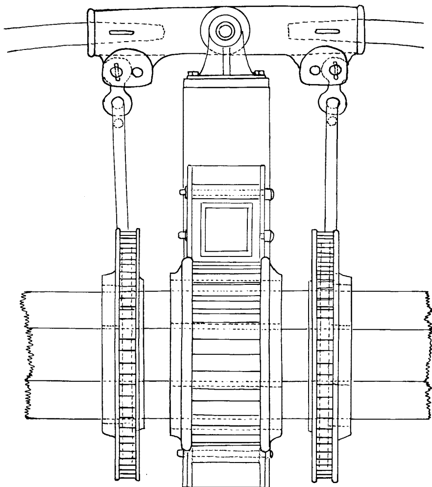
Fig. 14. J. G. Bergviks pumpspel
