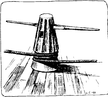
16. Gångspel från ett fynd av en Kogge från omkr. år 1400 - nära Bremen.
